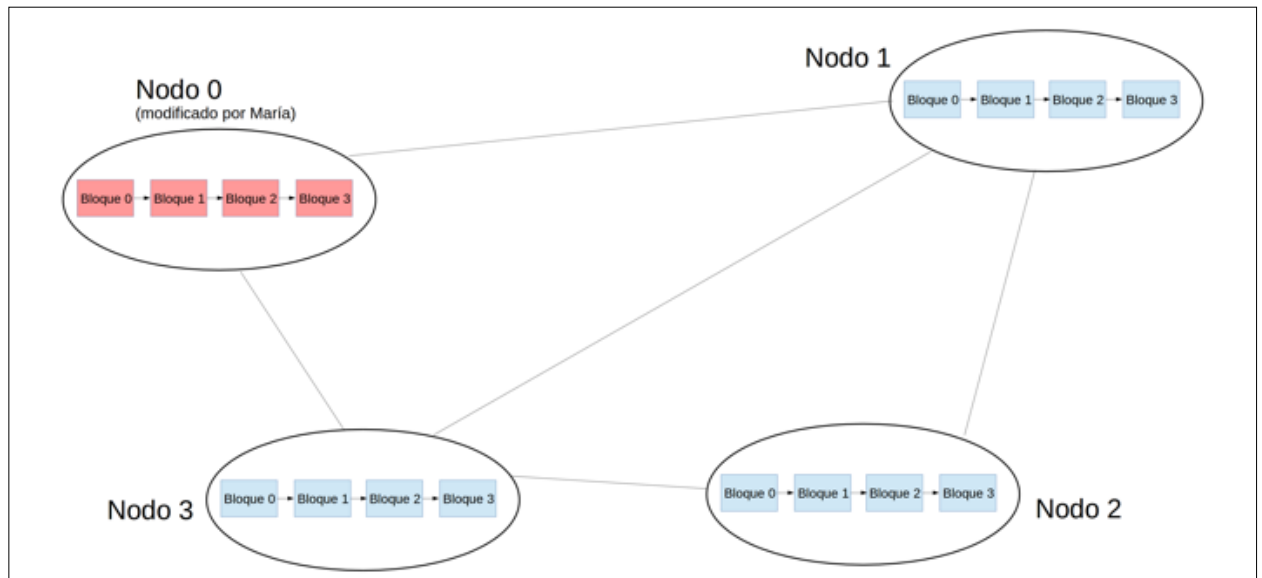
Figura 5: Blockchain distribuido a lo largo de diferentes nodos. Si María ha logrado modificar su propia copia del blockchain es fácil para el resto de la red detectar que dicho nodo no es coherente con el resto.
