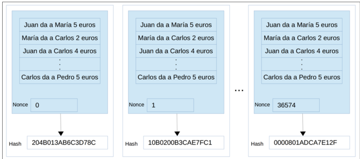
Figure 3: Un bloque con diferentes nonces y por tanto diferentes hashes. El bloque de la derecha contiene la característica deseada de 4 ceros al principio y se obtiene al probar el nonce 36574
