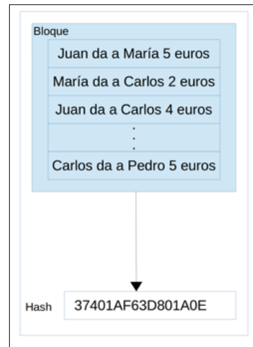
Figura 2: Un bloque y su respectivo hash
